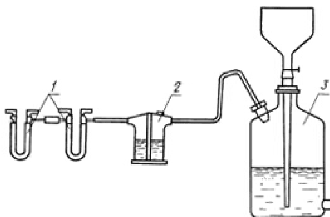
Установка для определения водяных паров
