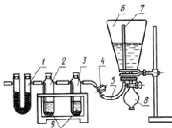
Установка для определения фосфористого водорода
