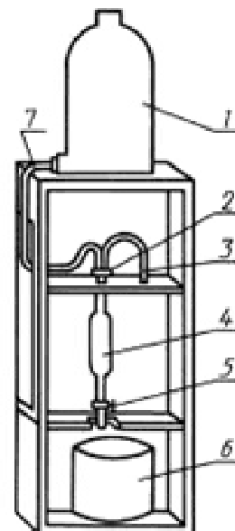
Установка для определения содержания воздуха и других малорастворимых в воде газов в ацетилене
